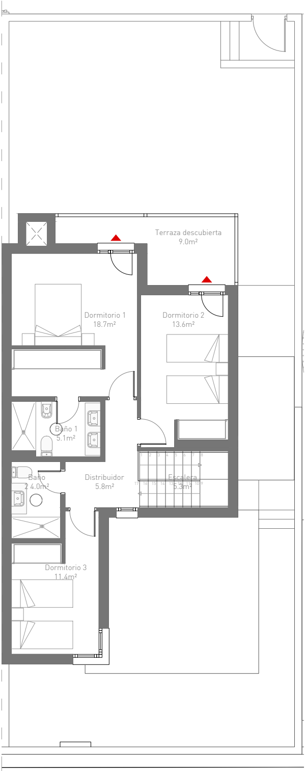
PLANTA PRIMERA
